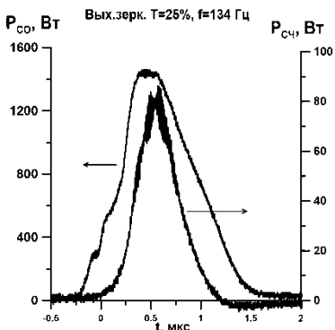
Рис. 1. Форма импульсов основных ( P_{\text{CO}} ) и суммарных ( P_{\text{сн}} ) частот
