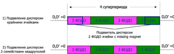
Рисунок 3 Принципиальная схема двух возможных вариантов подавления дисперсии для протонной опции коллайдера NICA
