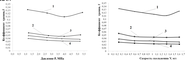
Рис. 1. Зависимость коэффициентов трения от давления (а) и скорости скольжения (б): 1 – сталь 12X13, 2 – (Ni-Cr-B-Si, Co-Cr-W-Ni-Si-B) 3- (Ni-Cr-B-Si, Co-Cr-W-Ni-Si-B) + 5 масс.% TiC, 4 - (Ni-Cr-B-Si, Co-Cr-W-Ni-Si-B) + 10 масс.% TiC
