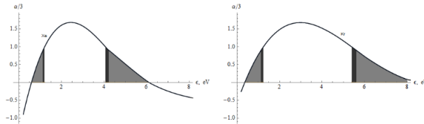
Рис.1. Значение параметра \alpha/3 от средней энергии фотоэлектронов для ксенона и криптона.
