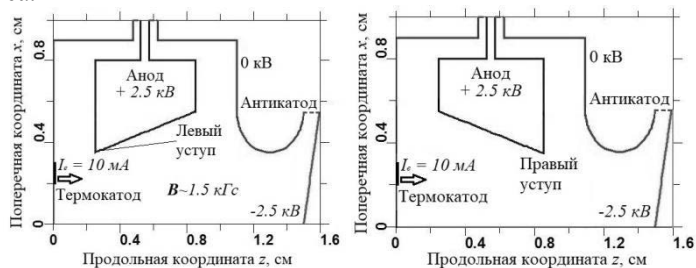
Рис. 1. Модели ионного источника Пеннинга в KARAT.
