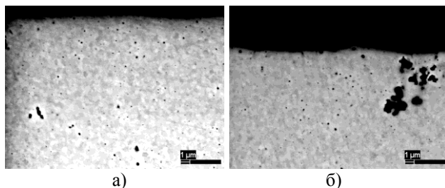
Рисунок 2 - Структура керамики диоксида циркония после лазерной обработки для разных мощностей лазерного излучения ( P_a < P_b ).
